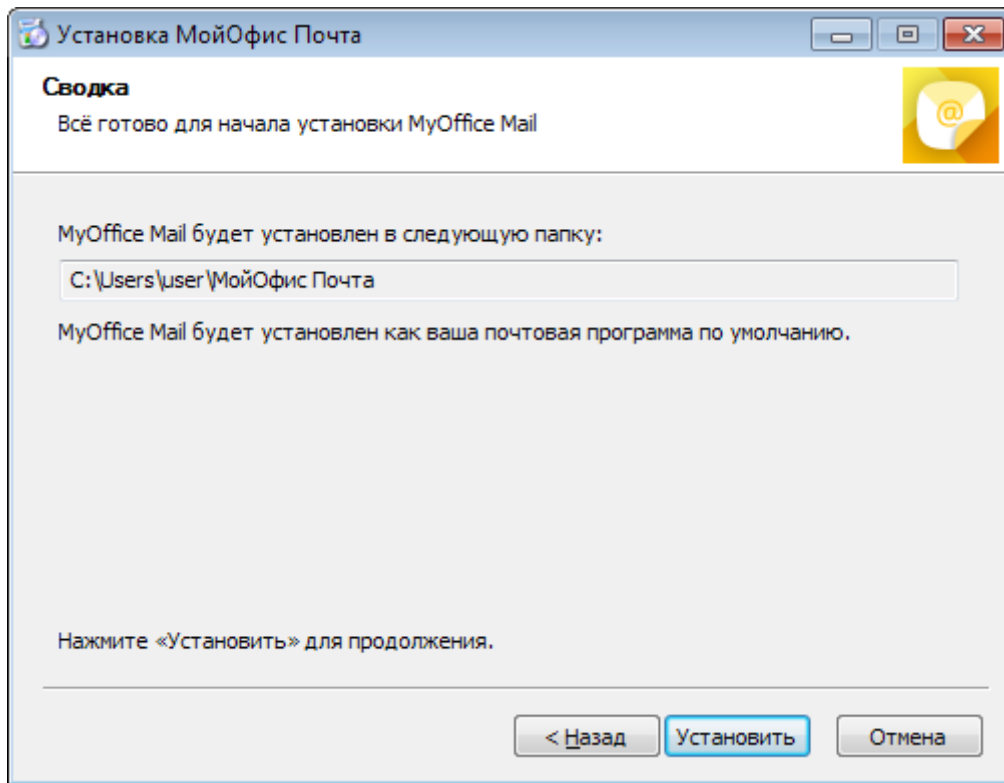
Рисунок 4 – Окно Сводка
