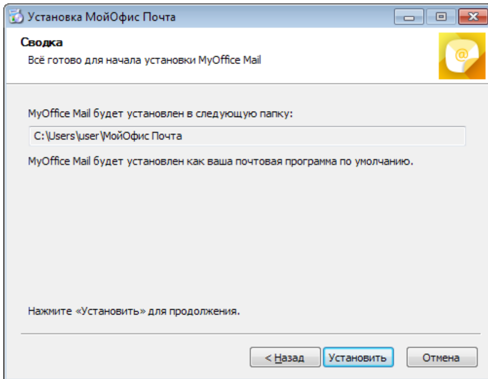
Рисунок 4 – Окно Сводка
