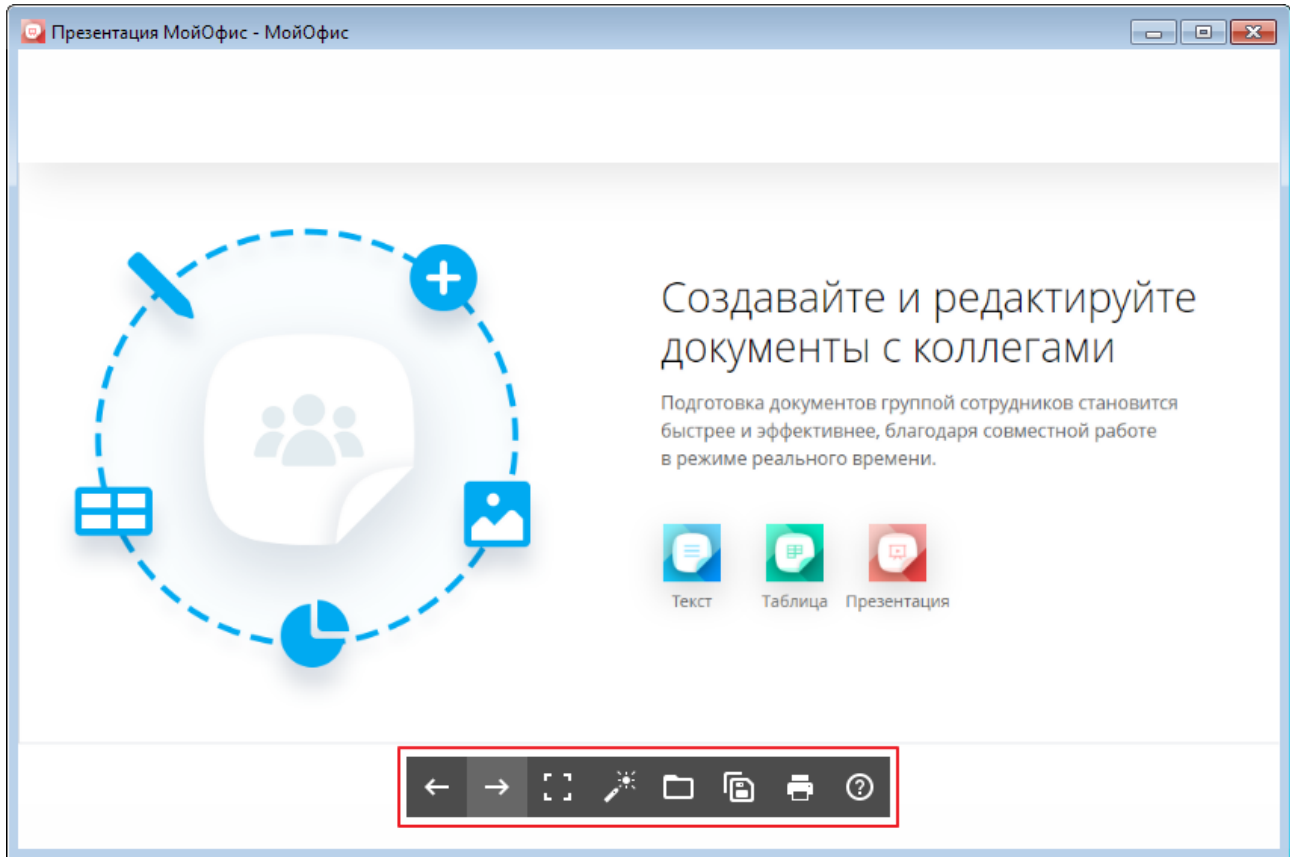
Рисунок 4 – Панель инструментов
